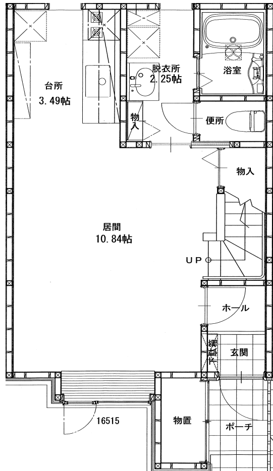
1F 間取り
